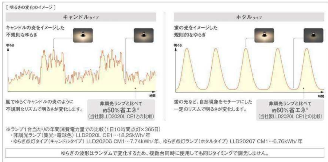
通常のLEDフラットランプと比較したゆらぎ点灯タイプの消費電力
