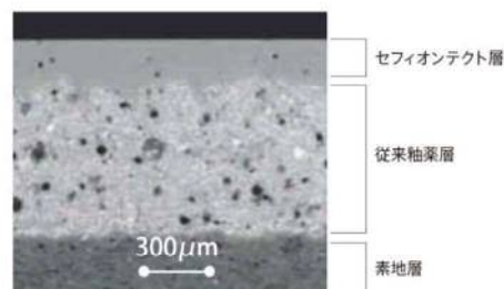
セフィオンテクト(新品) ※新品のセフィオンテクト便器の顕微鏡写真。 ※1μm=0.001mm
